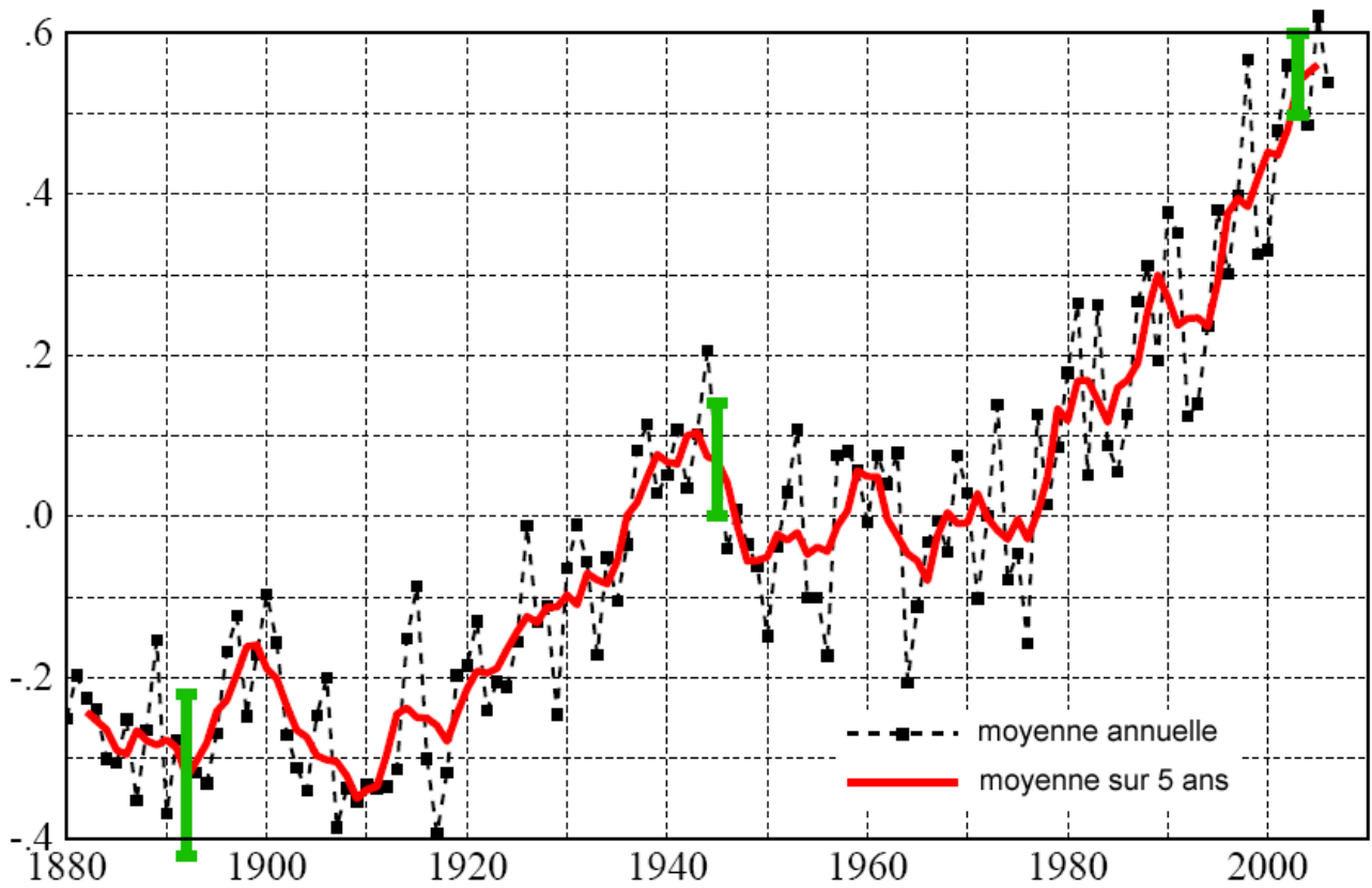
Évolution des températures moyennes mondiales sur mer et sur terre de 1880 à 2006. En ordonnée, se trouvent les écarts de températures en °C par rapport aux normales calculées pour la période 1951-1980.
